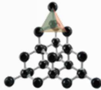
甲烷(正四面體) 鑽石(正四面體堆疊)
